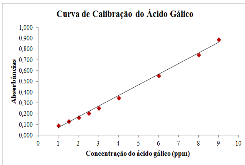
Figura 1 – Curva de Calibração do ácido gálico
